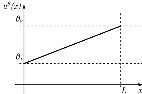
Figura 2.3: Soluzione stazionaria.
