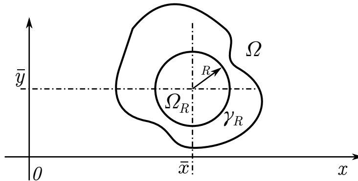
Figura 3.2: Circonferenza di frontiera \gamma_R .
